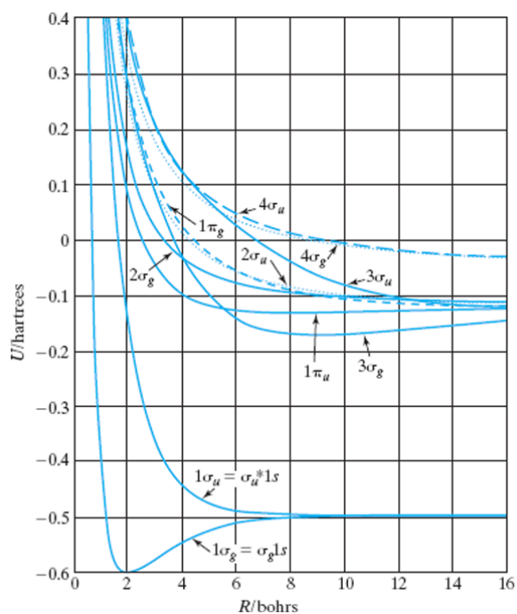
几个 \text{H}_2^+ 电子态的 U(R) 曲线。虚线用于帮助区分间隔较近的能级。在本图的尺度上无法观察到第一激发电子能级曲线在 12.5 bohrs 处的一个微小谷值，其势阱深度为 0.00006 hartrees。
